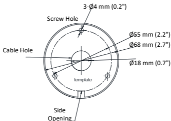
Рисунок 2-2 Шаблон крепления
