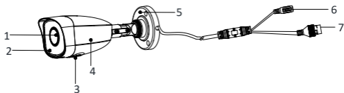
Рисунок 1-3 Внешний вид цилиндрической камеры типа III
